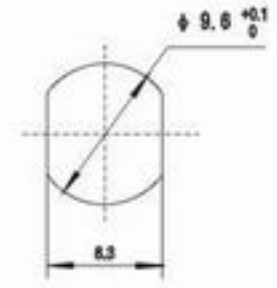
安装开孔尺寸 Mounting hole
