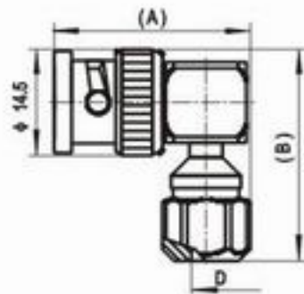
电缆剥线尺寸 Cable stripping dimensions
