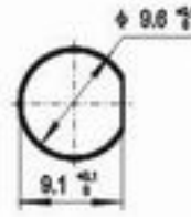
安装开孔尺寸 Mounting hole
